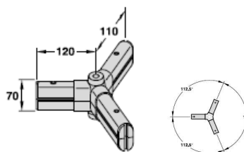
IDEA 400 型 45° Y 型连接件
