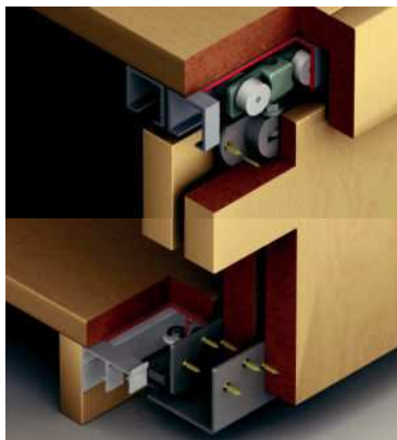
SILENT 60 嵌挂式推拉门五金, 三门用,最大承重 60kg
