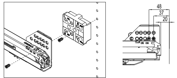
Distanzstück Innenschubkasten mit Holzblende / Spacer internal drawer with wood panel
