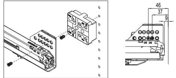
Distanzstück Innenschubkasten / Spacer internal drawer
